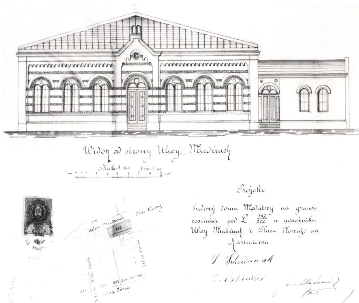
Ryc. 13. Bejt ha-midrash Bne Emuna, projekt Jacka Matusińskiego, zatwierdzony 29 marca 1886 r.: elewacja północna i plan sytuacyjny; w zasobie ANK, sygn. Dz. VIII, l.s. 358
