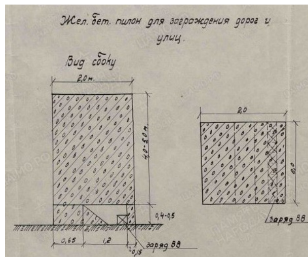
Sowiecki szkic przedstawiający budowę niemieckich słupów przeciwpancernych; w zasobie Centralnego Archiwum Ministerstwa Obrony Federacji Rosyjskiej (CAMO FR), fond 236, opis 2673, dzieło 2778, s. 39
