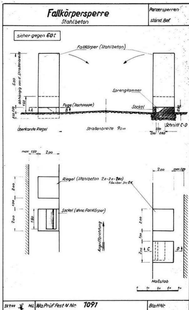
Niemiecki rysunek przedstawiający budowę niemieckiej zapory przeciwpancernej ( Fallkörpersperre ); w zbiorach prywatnych
