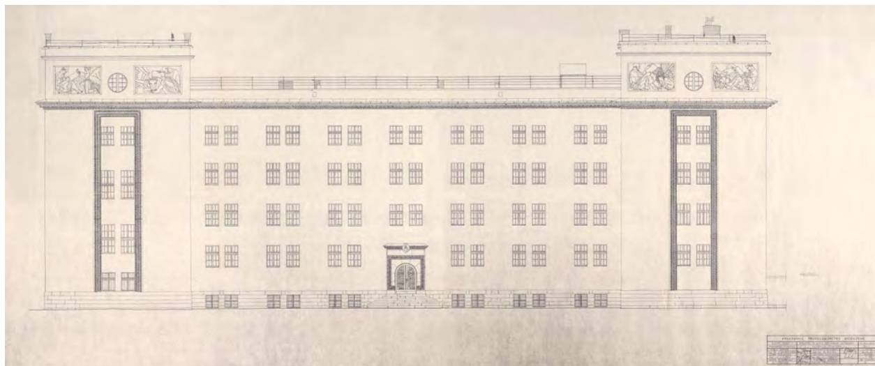
Inwentaryzacja fasady wschodniej gmachu Śląskiego Seminarium Duchownego w Krakowie, 1979; w zasobie ANK, Krakowskie Przedsiębiorstwo Geodezyjne, sygn. 29/1406/1168
