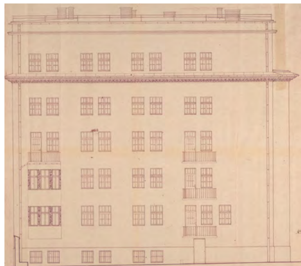
Inwentaryzacja fasady południowej gmachu Śląskiego Seminarium Duchownego w Krakowie, 1979; w zasobie ANK, Krakowskie Przedsiębiorstwo Geodezyjne, sygn. 29/1406/1168
