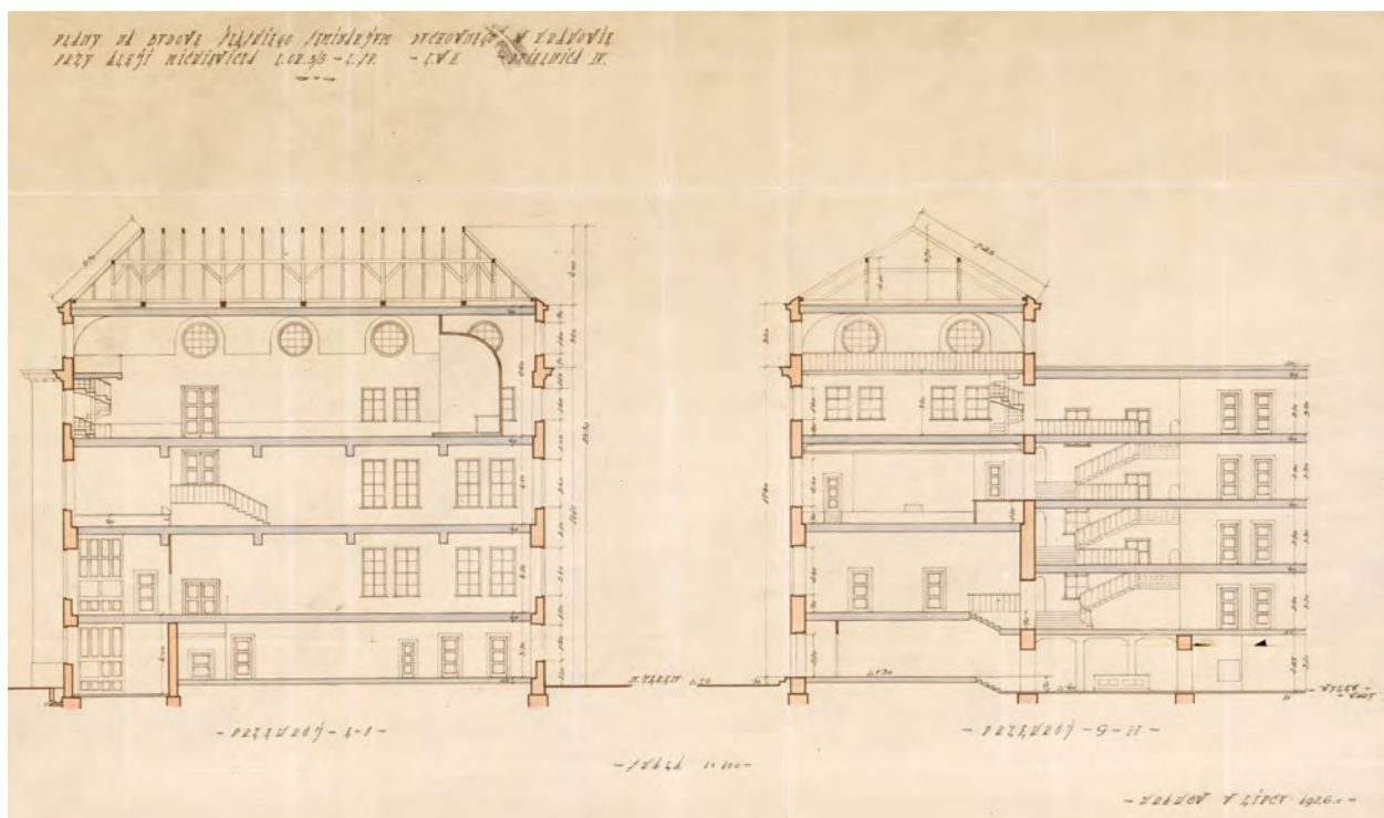
Projekt pierwotny z czterospadowymi dachami skrzydeł, Plany na budowę Śląskiego Seminarium Duchownego w Krakowie przy Alei Mickiewicza L. or. 3/5-L.Sp-L.W.H.- Dzielnica IV, Zygmunt Gawlik, lipiec 1926 r.; w zasobie AAdK, ASDKr, sygn. 47/1133, s. 10 v.
