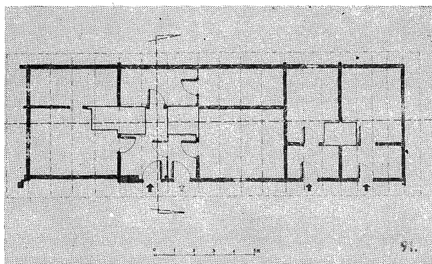
Rzut poziomy chaty przy ul. Mazowieckiej nr 51, (zb. IHAiKZ PK) (il. 28/91)
