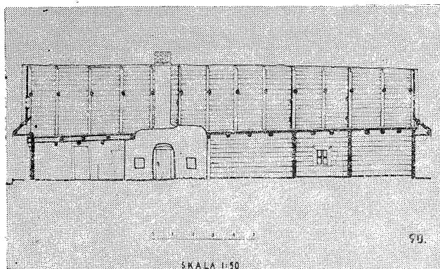
Przekrój podłużny chaty przy ul. Mazowieckiej 51 na Krowodrzy z jednym kominem „na dwie strony”, charakterystycznym dla wsi otaczających dawny Kraków, stan z 1958 r. (zb. IHAiKZ PK) (il. 29/90)
