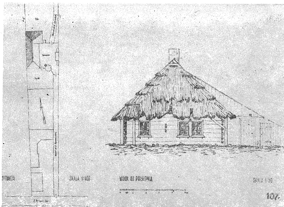
Dom przy ul. Mazowieckiej nr 37, zagospodarowanie działki i widok od strony południowej. Widoczna mieszana konstrukcja ścian z charakterystycznym przystępem. (zb. IHAiKZ PK). (il. 27/107)
