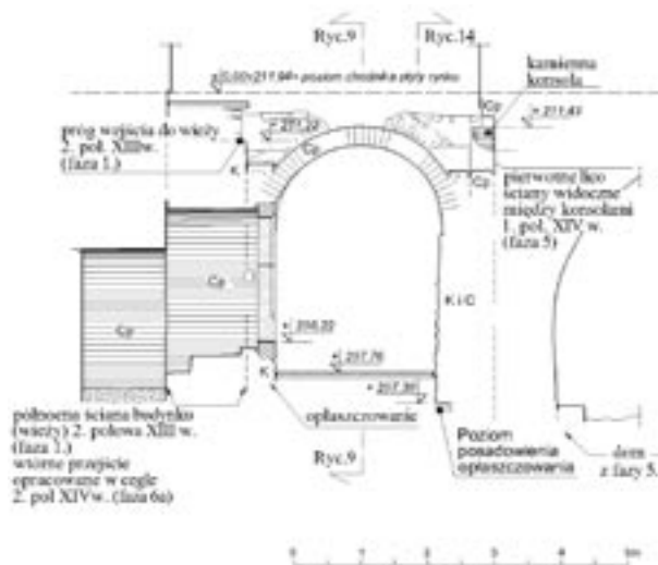
Ryc. 6. Przekrój poprzeczny przez korytarz 007
