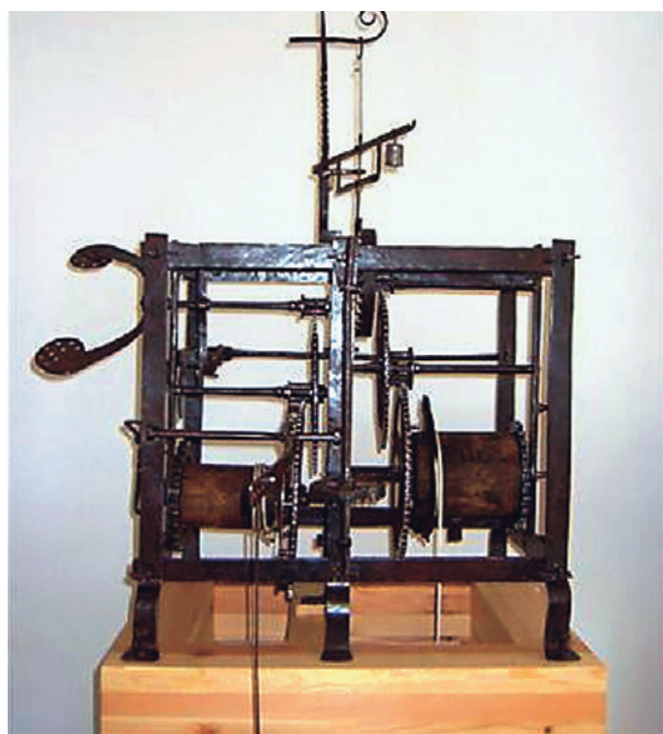
Ryc. 6. Mechanizm zegara z oratorium klasztoru ss. Norbertanek w Żukowie koło Gdańska, poł. XVII w. – rzadki i niezwykle cenny ze względu na zachowany pierwotny regulator kolebnikowy: a) widok od strony wychwyty, b) widok na stabilizator bicia tzw. wiatrak (lewa strona), Muzeum Historyczne Miasta Gdańska, oddział Muzeum Zegarów Wieżowych, depozyt
