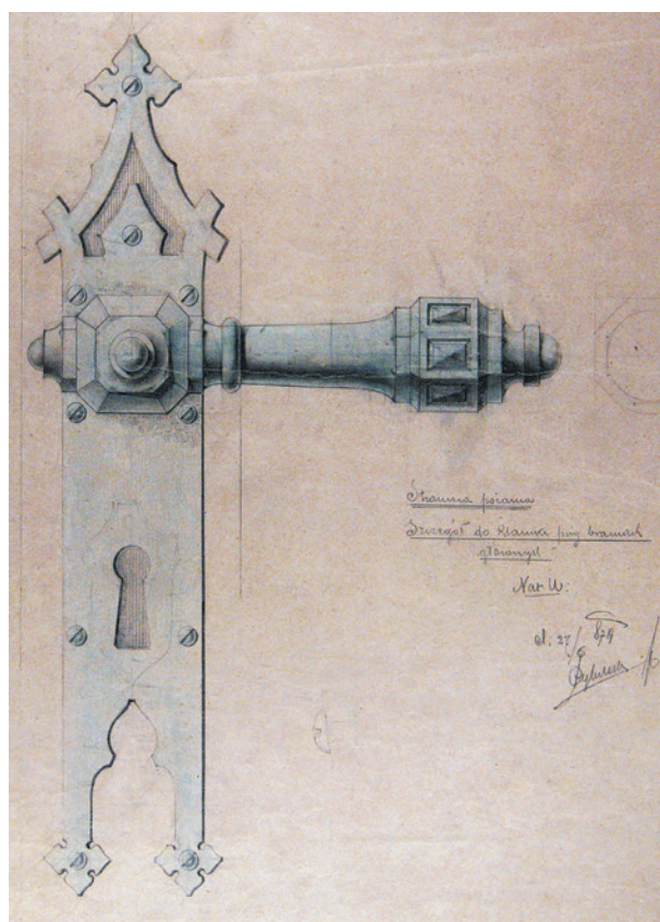
Projekt wykonawczy klamki do głównej bramy w koszarach Miejskiej Straży Pożarnej przy ul Kolejowej z 27 czerwca 1879 r., sygnowany przez J. Cybulskiego; APKr, sygn. ABM, Teka XXXI, plan 80
