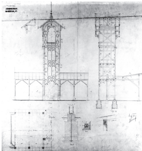
Projekt wykonawczy otwartej wiaty i pierwszej drewnianej wspinalni z 19 maja 1879 r., sygnowany przez J. Cybalskiego; wł. APKr, sygn. ABM, Teka XXXI, plan 75
