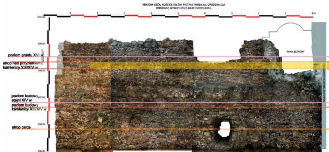
5. Rejestracja badań archeologicznych po wschodniej stronie kościoła św. Piotra i Pawła: ujawniona elewacja budynku wpisanego w siatkę modułową Około z czasów Władysława Łokietka; opr. pod kierunkiem Jacka Poleskiego z udziałem Agaty Kuci i Jakuba Nawrota
