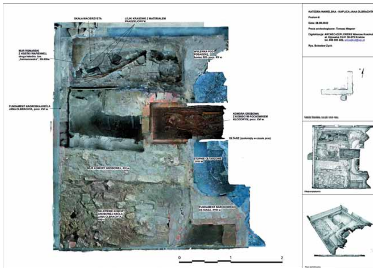
1. Archikatedra na Wawelu, kaplica grobowa króla Jana Olbracht, odkrycia pod posadzką; inwentaryzacja i interpretacja odkryć, opr. Tomasz Wagner, firma archeologiczna Archeo-Explorers Wiesław Koszkuł, Bolesław Zych
