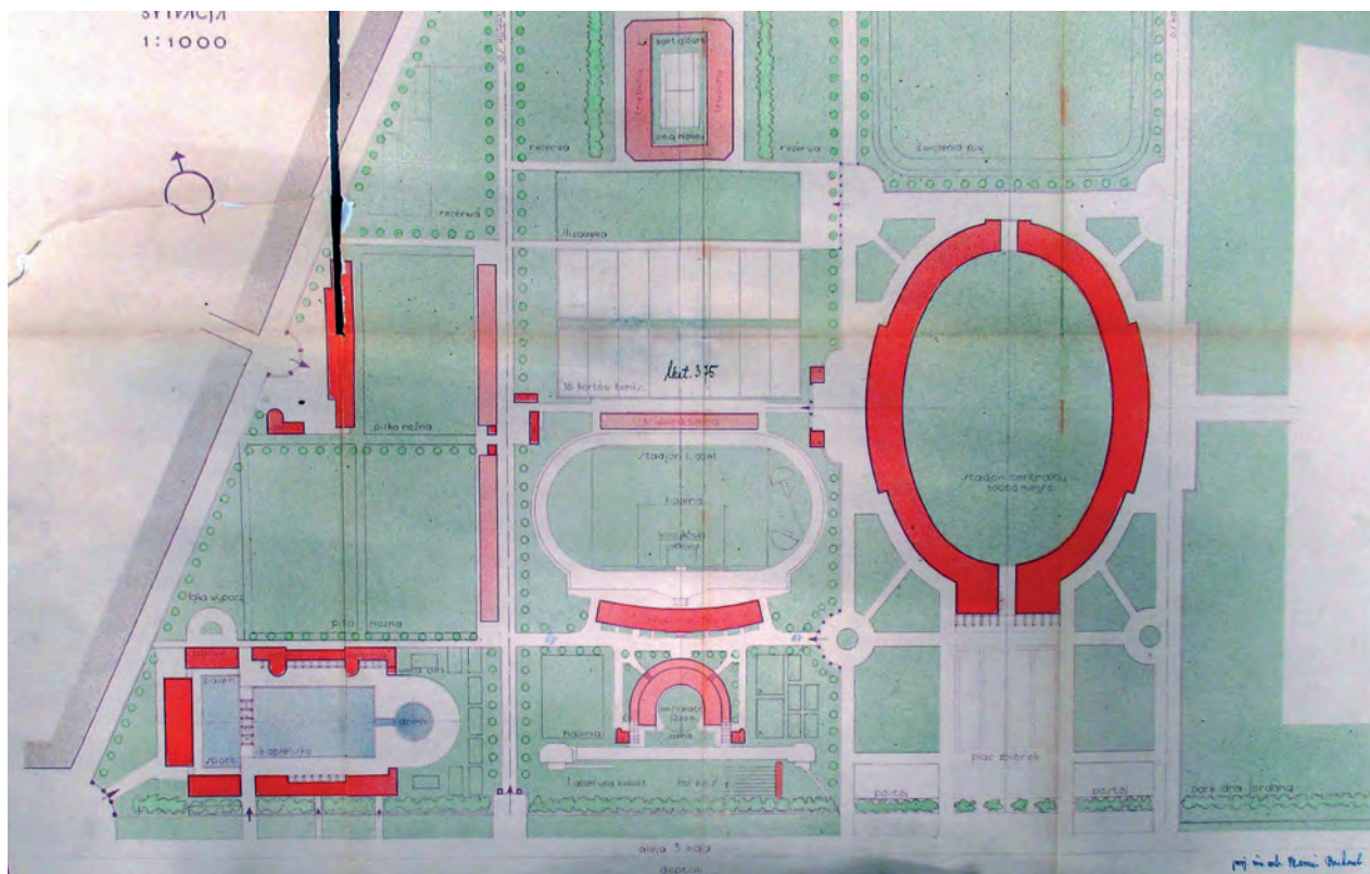
21. Miejski Stadion Sportowy przy Błoniach, al. 3 Maja, 1933, projekt arch. Marcin Bukowski, Archiwum Narodowe w Krakowie, sygn. 29/1410/ABM/TAU BUP 1
