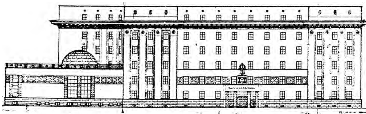
19. Projekt Domu Akademickiego UJ, al. 3 Maja 5, 1924, arch. Wacław Krzyżanowski, za Maria Jolanta Żychowska, Między tradycją a awangardą. Problemy stylu w architekturze Krakowa lat międzywojennych , Kraków 1991
